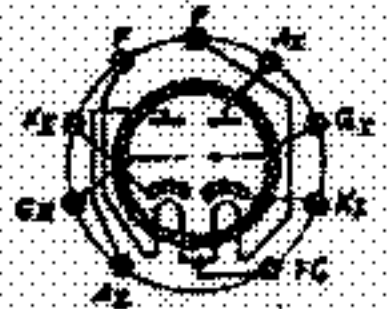
ECC 81
