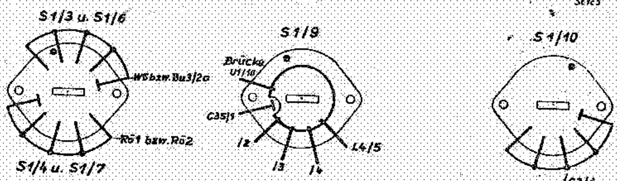
Außenseiten der Schaltebenen nach Montage im HF-Baustein
